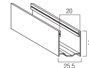
Guida in alluminio A27 GUIAL..27M 25,5 x 30 mm
